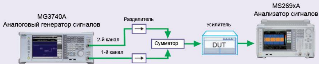
Схема подключения для оценки интермодуляционных характеристик усилителя
