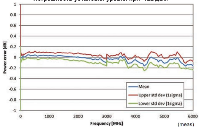
Частотная характеристика
